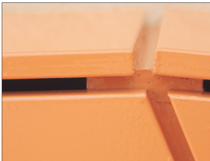
Afbeelding 1. Voorbeeld van goed afronden, ventileren en dilateren van plaatmateriaal.
