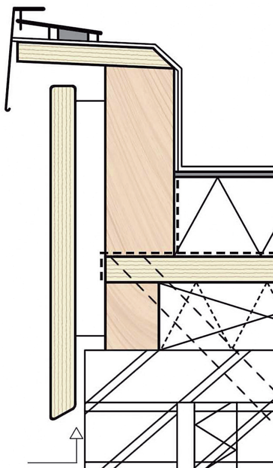
Figuur 8. Voorbeeld aanbrengen van een boeiboord
