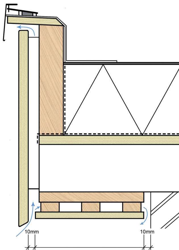
Figuur 9. Voorbeeld uitvoering van een dakoverstek
